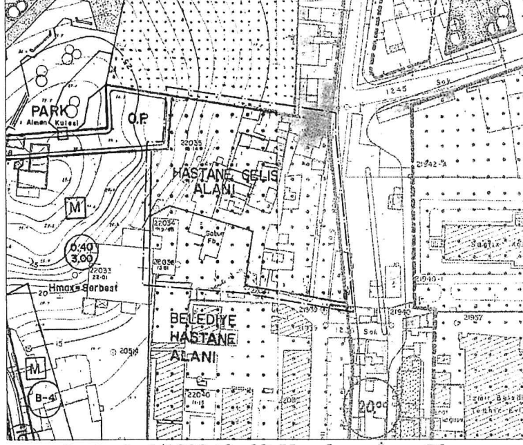
Resim 3: 1/1000 ölçekli Uygulama İmar Planı
